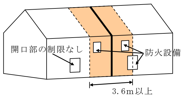
(立面図)
