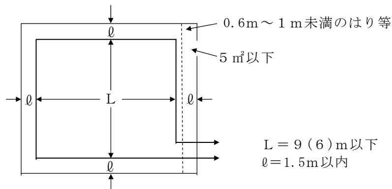
第11-32 図 差動式分布型（空気管式）
