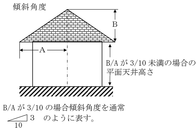
傾斜天井の角度、面積、平均高さの出し方
